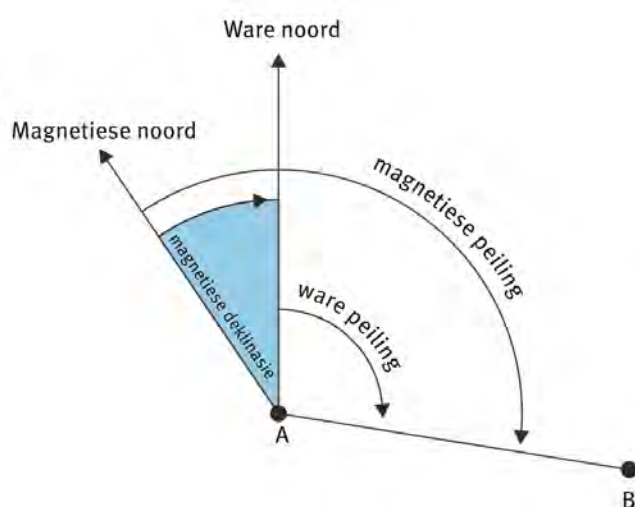
Figuur 5 Ware noord, magnetiese noord en ware peiling
